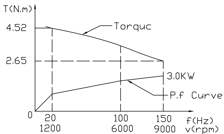
扭矩/功率曲线
