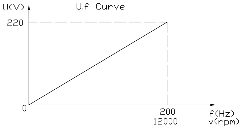
频压曲线
