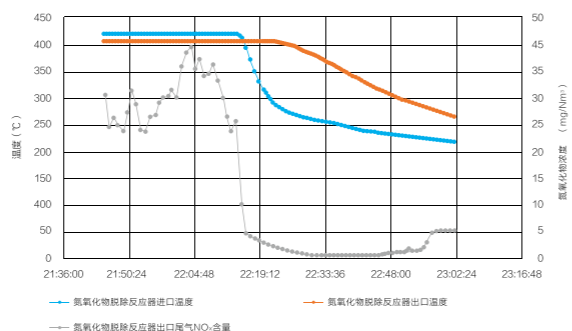
图5 氨氧化物脱除反应器通氨延长至35分钟后的测试结果
