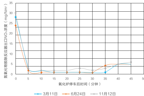
图6 改进后停车过程氨氧化物脱除反应器出口尾气 NO x 含量变化
