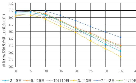
图4 氨氧化炉停车后氨氧化物脱除反应器出口温度变化
