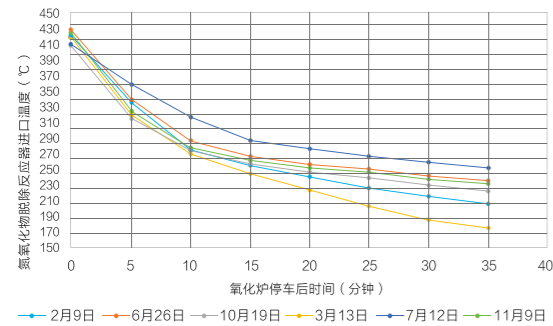
图2 氨氧化炉停车后氨氧化物脱除反应器进口温度变化
