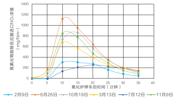
图3 氨氧化炉停车后氨氧化物脱除反应器出口尾气 NO x 含量变化
