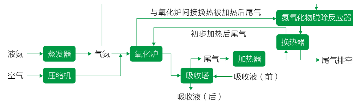
图1 氨氧化系统流程简图
