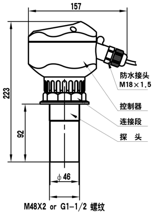
M48×2 或 G1-1/2 螺纹传感器
