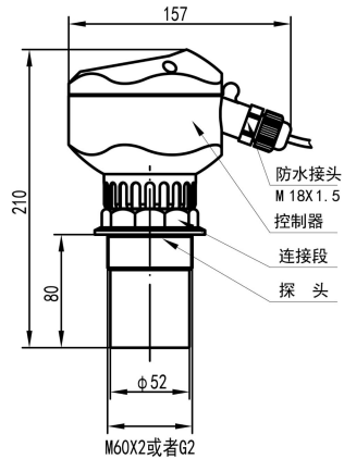
M60×2 或者 G2 螺纹传感器
