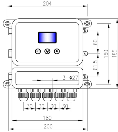
结构图
