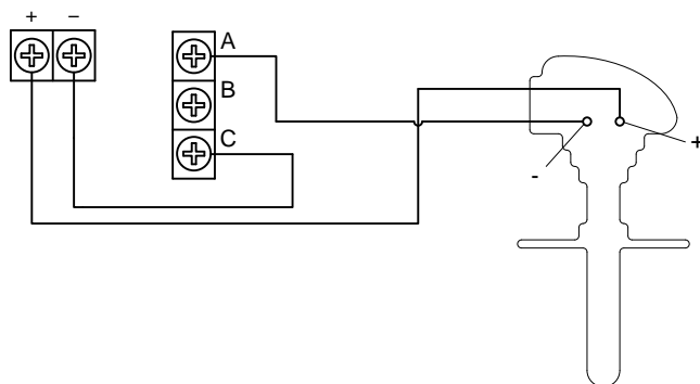
两线制变送器配电接线
