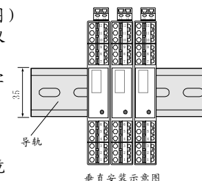
垂直安装示意图
