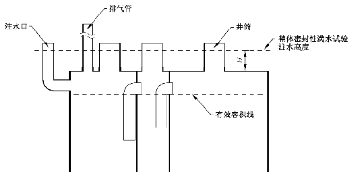
图 B.1 三格化粪池密封试验示意图
