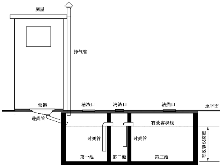
图 A.1 农村三格式户厕构造示意图
