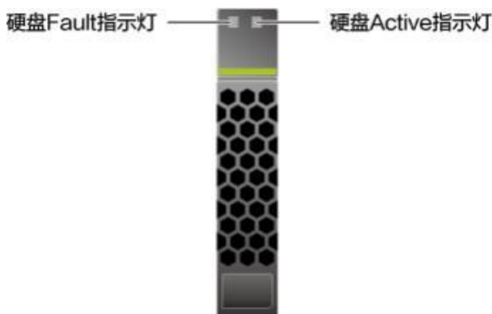
图 2-8 SAS/SATA 硬盘指示灯
