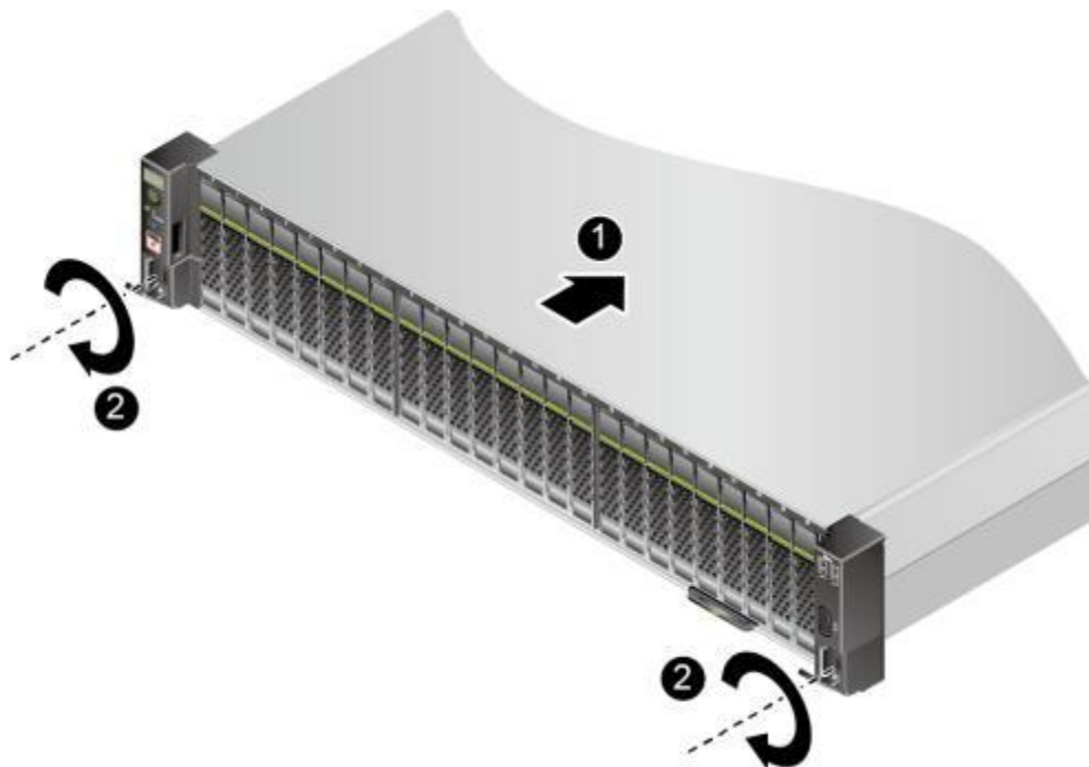
图 5-9 安装服务器
