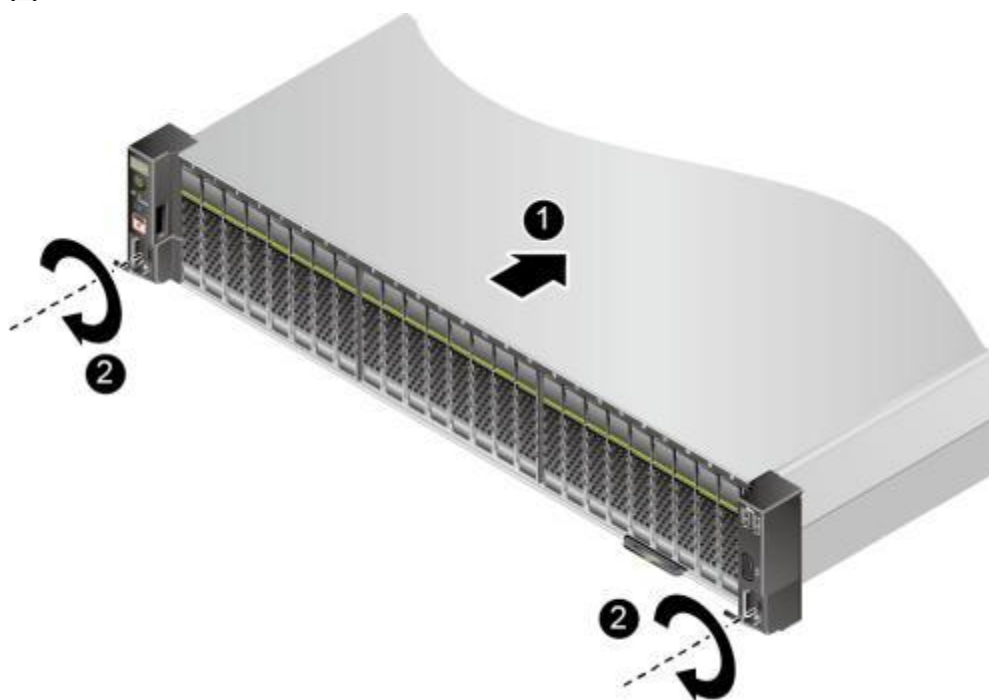
图 5-7 安装服务器
