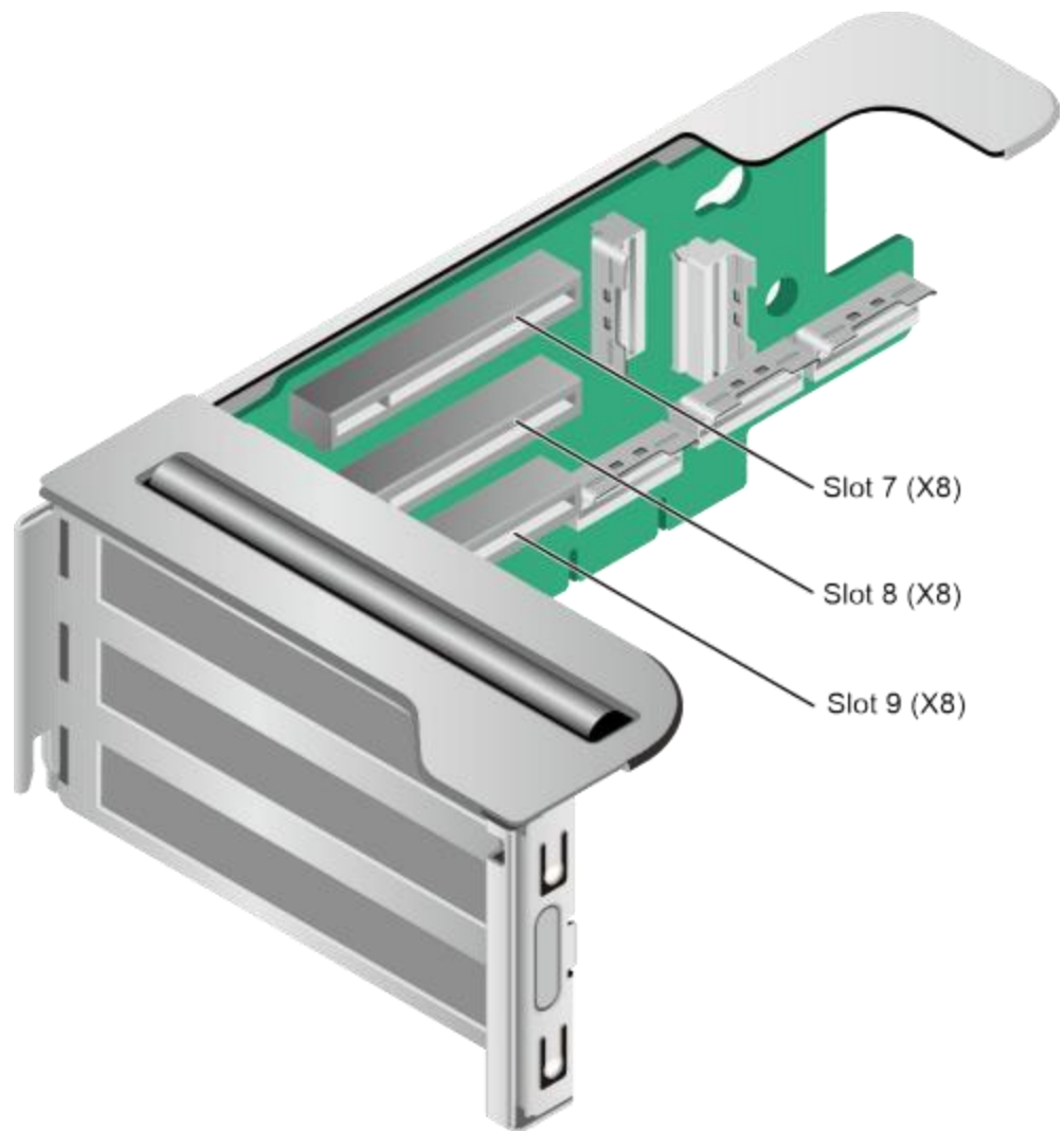
图 2-17 Riser 卡 2
