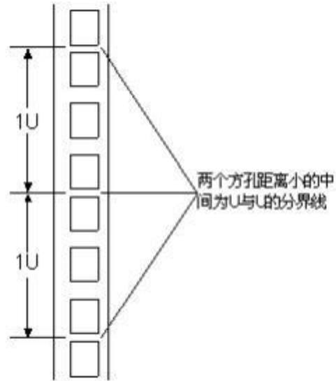
图 5-4 机柜导槽 U 与 U 的间距区分示意图
