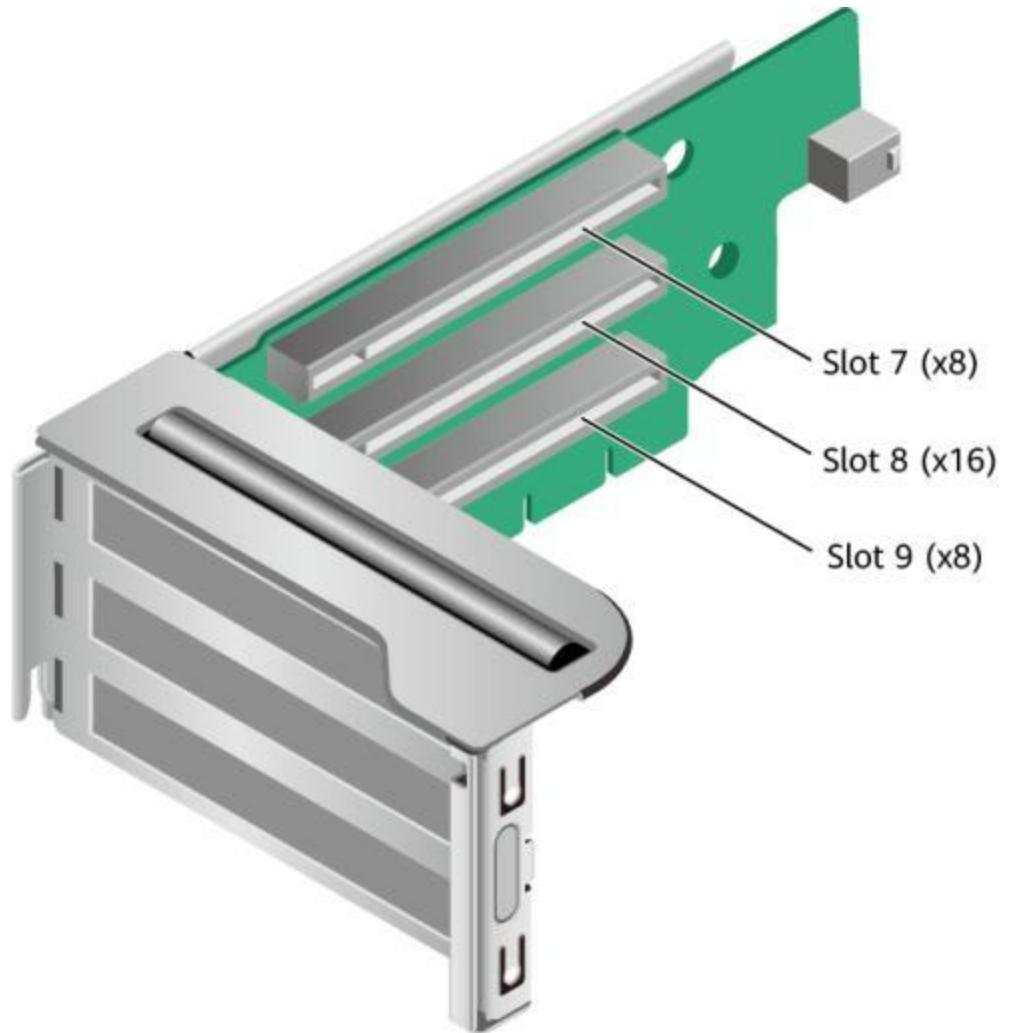
图 2-10 Riser 卡 2
