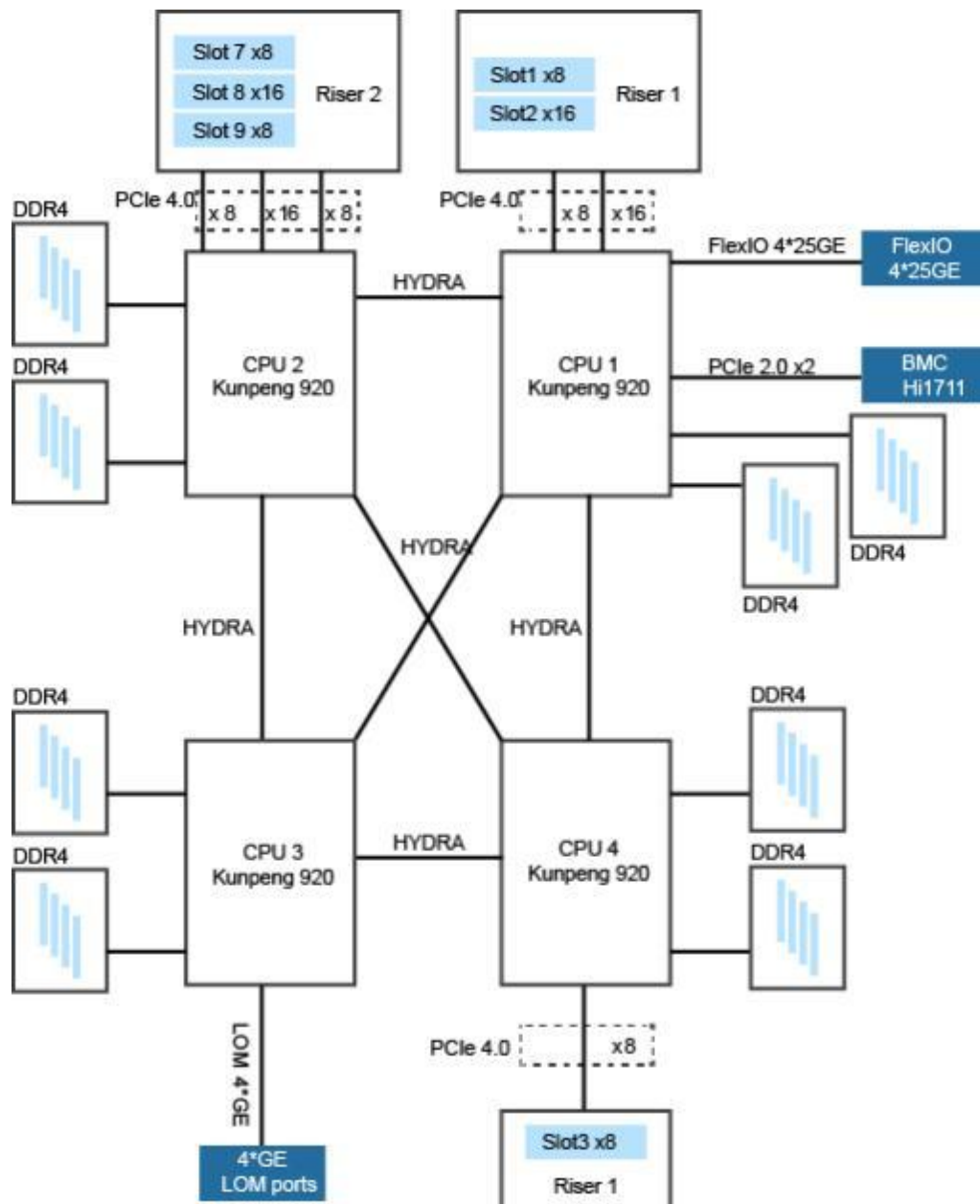
图 1-3 逻辑结构
