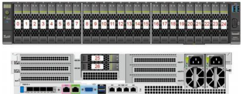
图 2-7 25x2.5 英寸硬盘 EXP 配置硬盘编号
