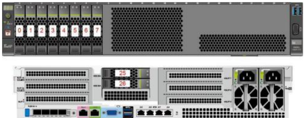
图 2-6 8x2.5 英寸硬盘配置的硬盘编号
