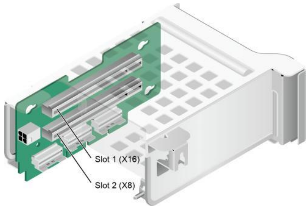
图 2-16 Riser 卡 1
