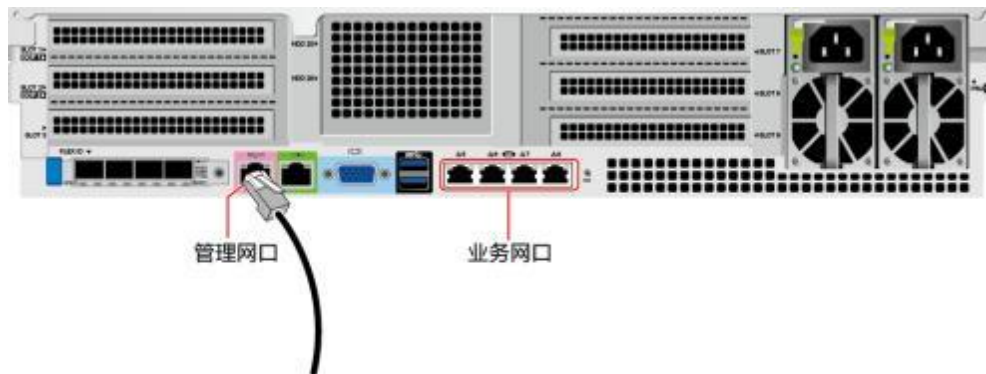
图 5-11 连接网线
