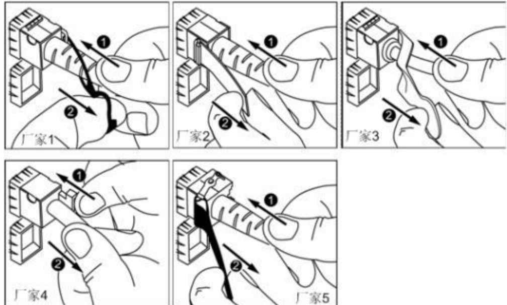
图 5-13 拔出 SFP+电缆
