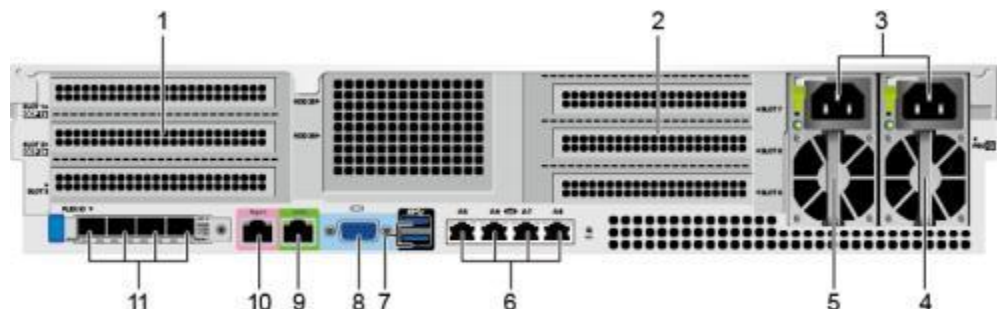
图 2-3 后面板组件
