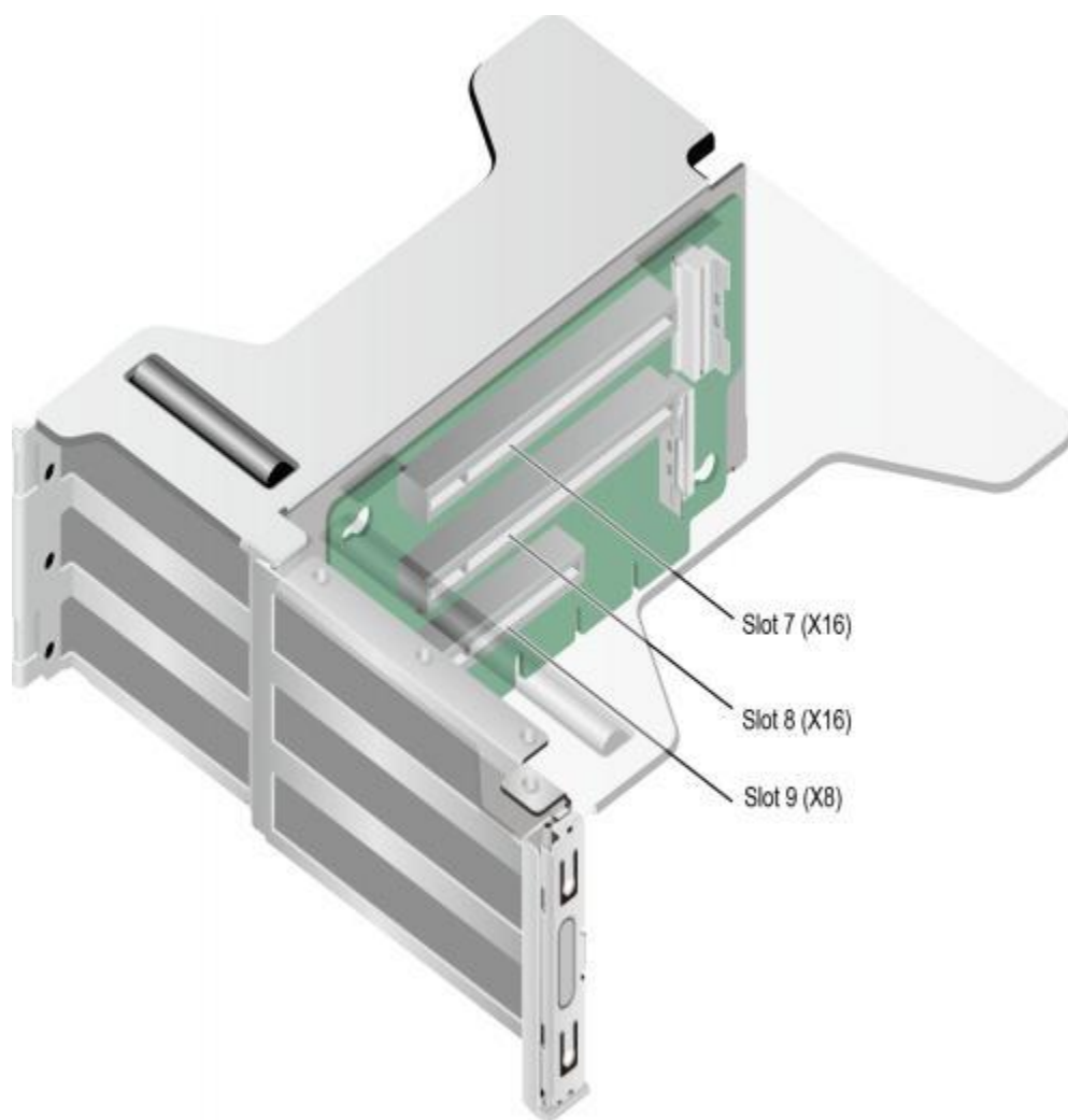
图 2-14 Riser 卡 2-2
