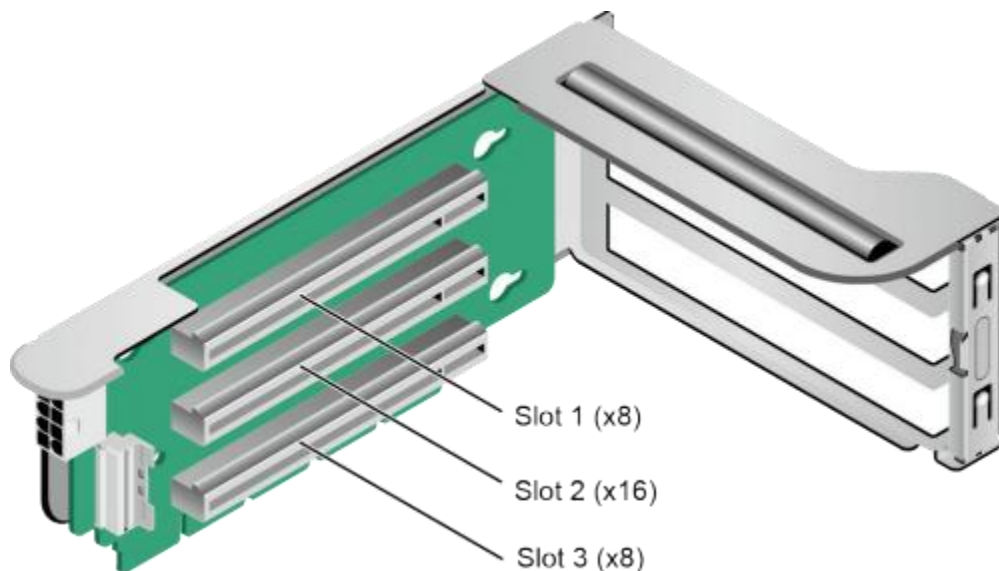
图 2-12 Riser 卡 1
