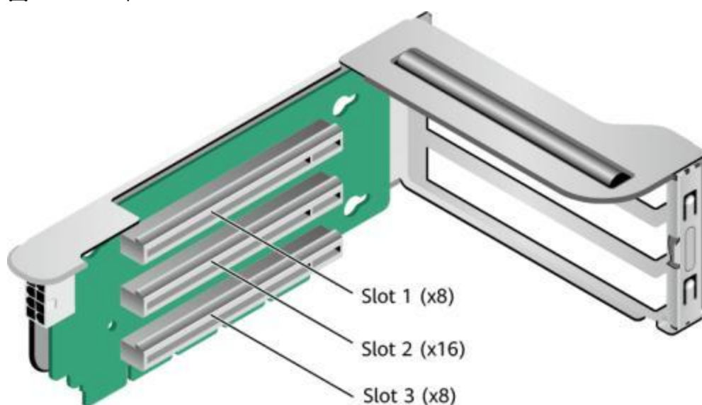
图 2-9 Riser 卡 1
