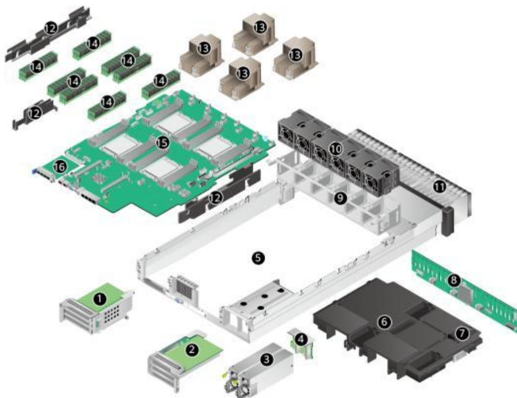
图 1-2 部件
