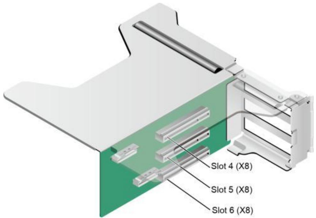
图 2-13 Riser 卡 2-1
