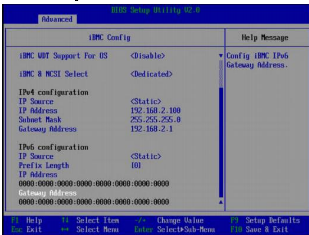
图 5-21 iBMC Conig 界面 2
