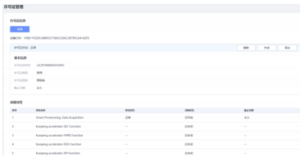
图 5-66 许可证管理
