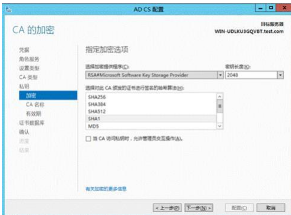
图 7-18 CA 的加密
