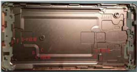
机加工件各台阶面的段差测量
