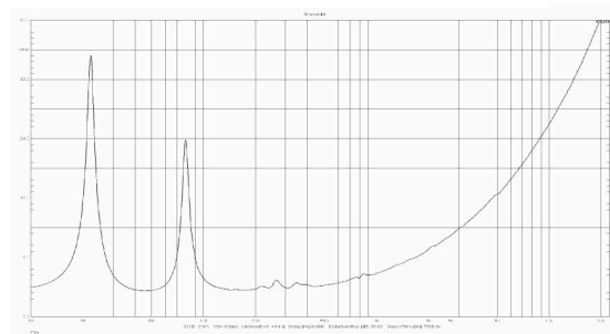
阻抗曲线
