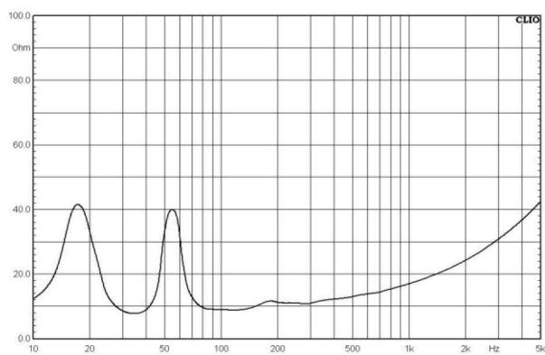
阻抗曲线
