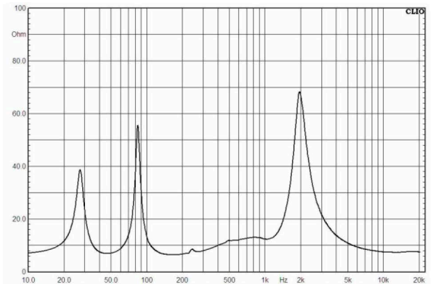
阻抗曲线
