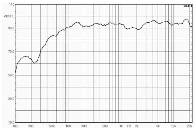
频响曲线
