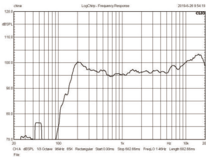
频响曲线
