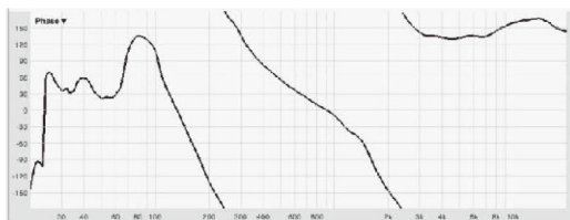
相位曲线
