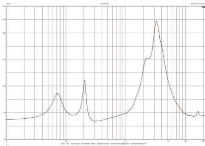
阻抗曲线
