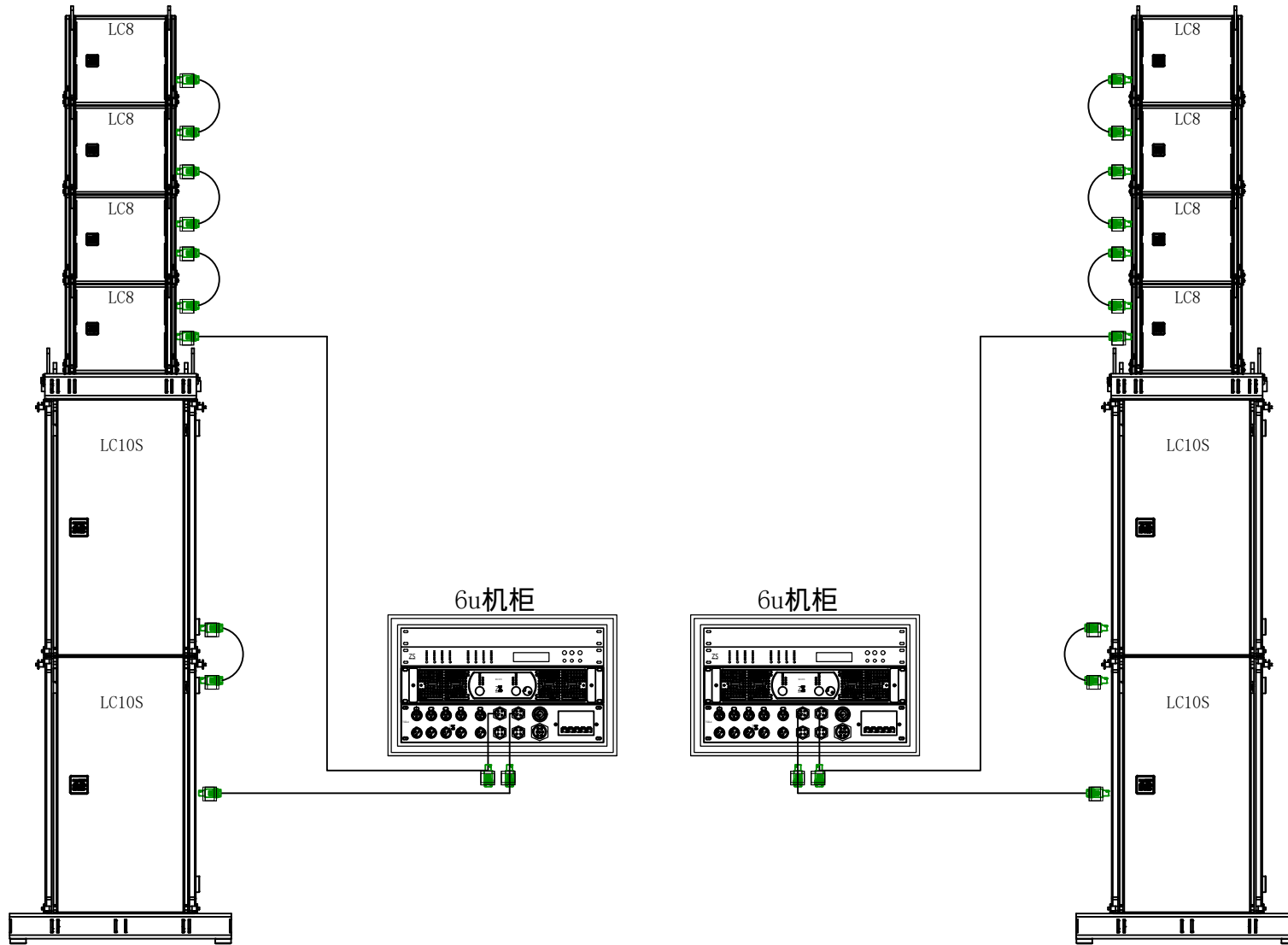
ZSOUND LC8+LC10S 8+4堆叠连线图
