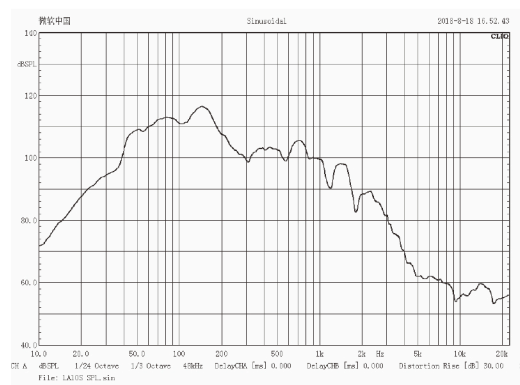
频响曲线
