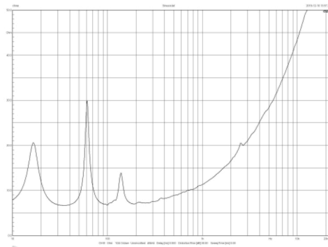
阻抗曲线
