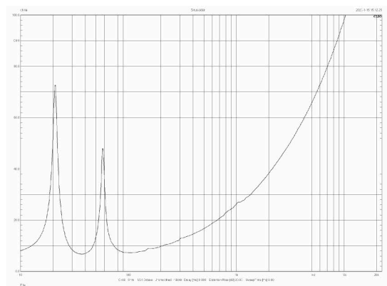
阻抗曲线
