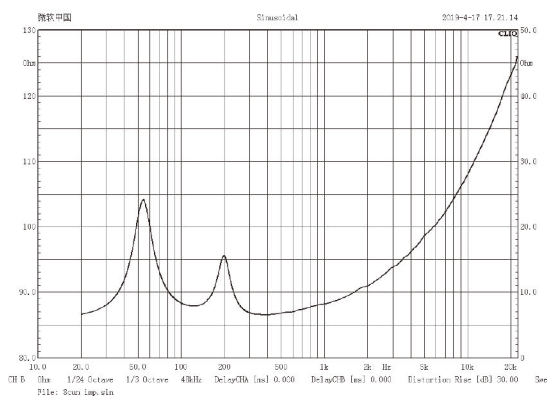
阻抗曲线
