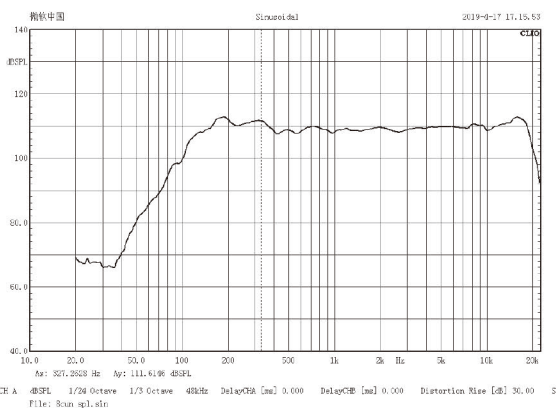
频响曲线
