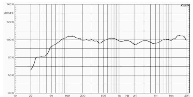
频响曲线
