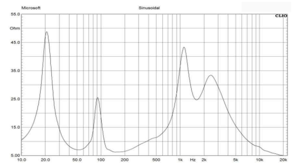
阻抗曲线
