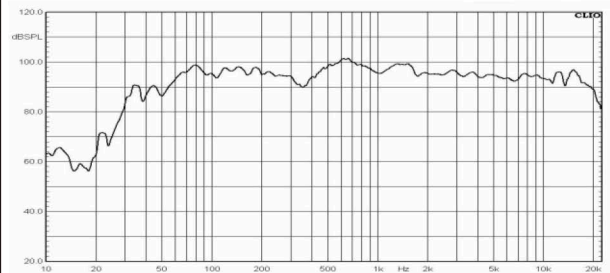
频响曲线
