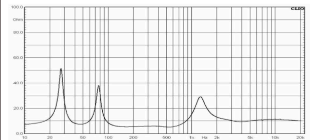
阻抗曲线
