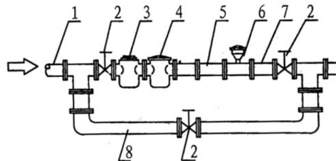
图4 系统配置图
