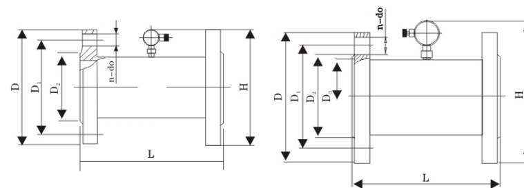
图3 法兰连接结构
