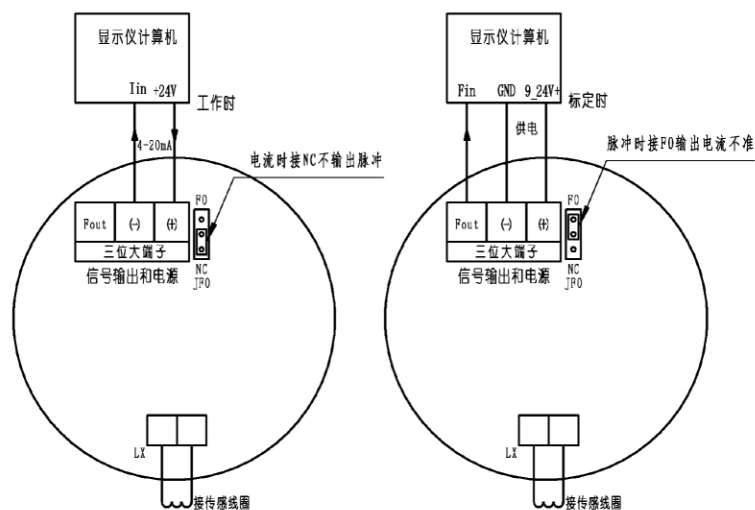
附录2: TB2WE 二线制涡轮流量计接线图
