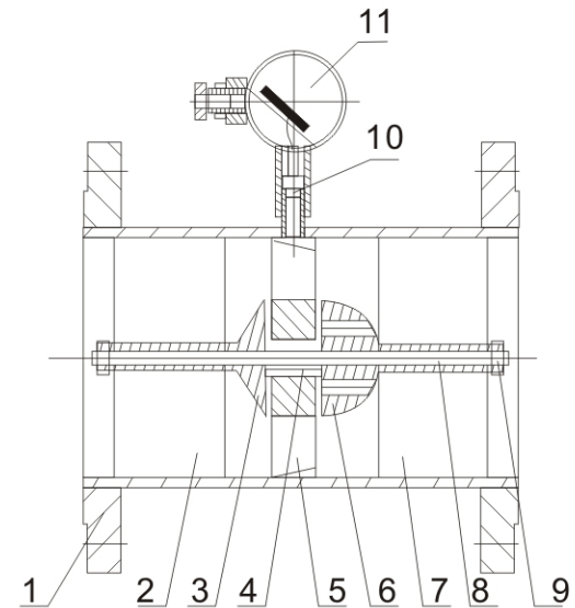
1.壳体 2.导流体 3.椎体 4.轴承系统 5.叶轮 6.反推体 7.导流件 8.长轴 9.螺母 10.信号检测器 11.放大器
