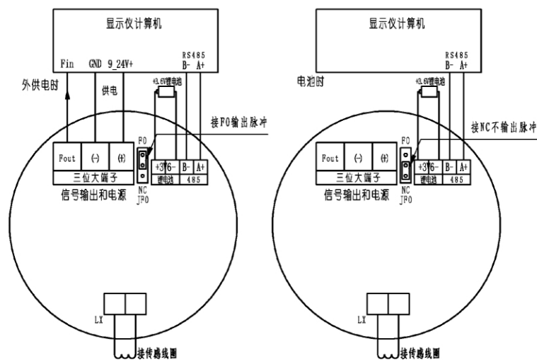
附录3: TB3WE 三线制涡轮流量计接线图
