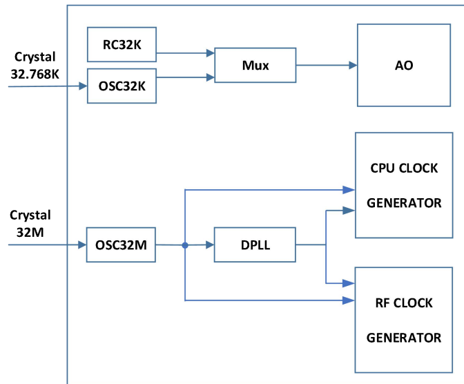
图 3-1 系统时钟
