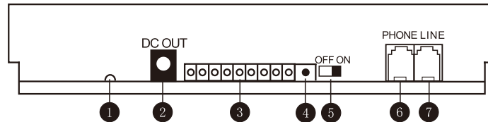
报警主机后面板
