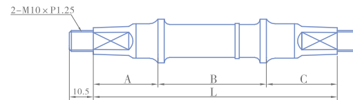
Nut Type
