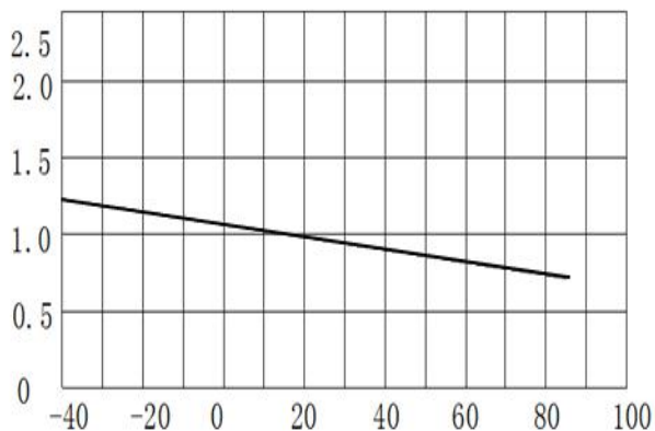
亮度与环境温度关系曲线图
