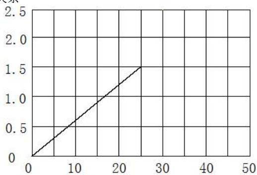
亮度与正向电流关系曲线图
