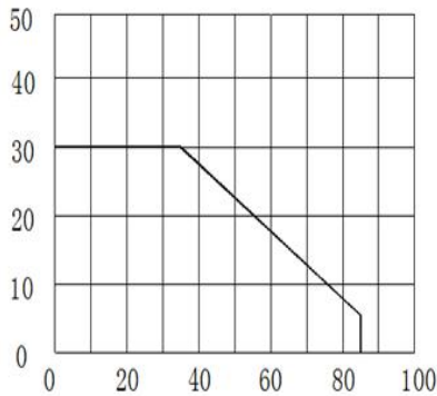
正向电流递减曲线图
