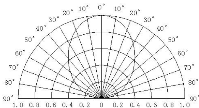
发光角度图解
