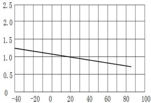
亮度与环境温度关系曲线图
