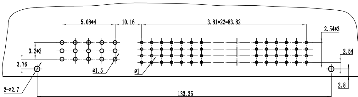
插头推荐安装开孔尺寸
