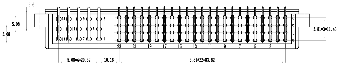
插头推荐安装开孔尺寸
