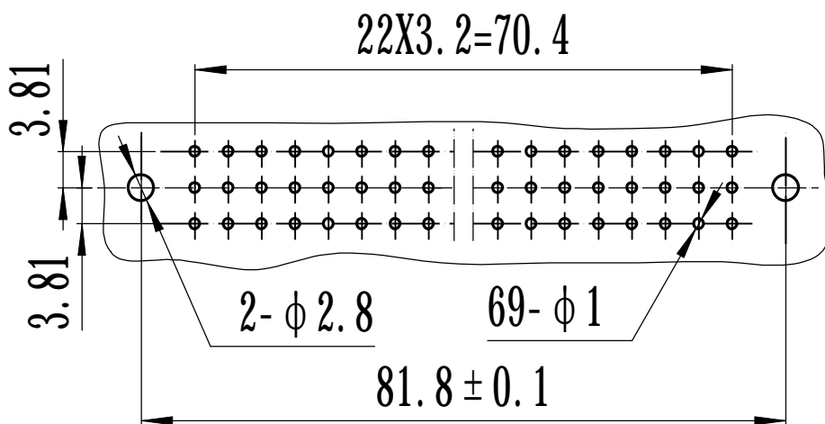
插座安装开孔尺寸
