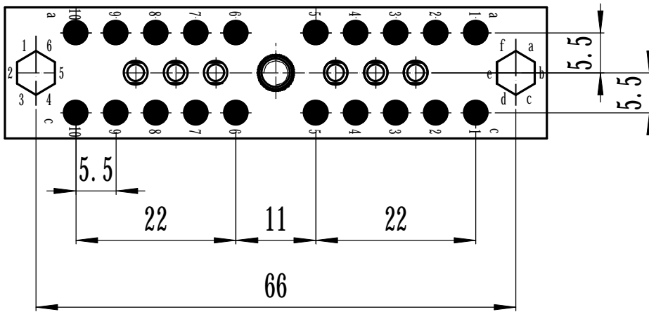
插座安装开孔尺寸
