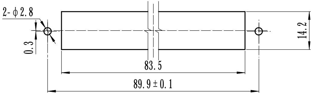
插座安装开孔尺寸
