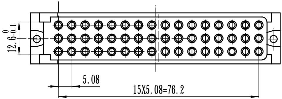
插座安装开孔尺寸
