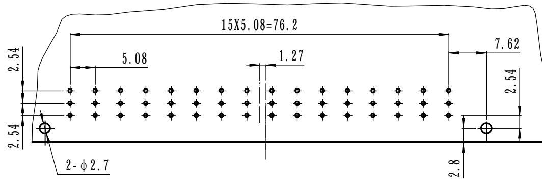
插头推荐安装开孔尺寸
