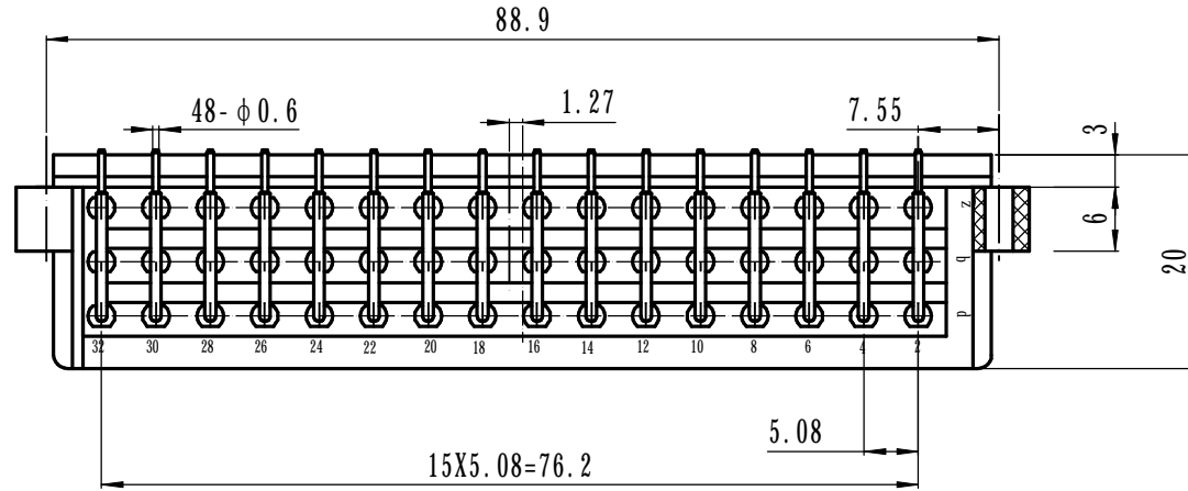
插头推荐安装开孔尺寸
