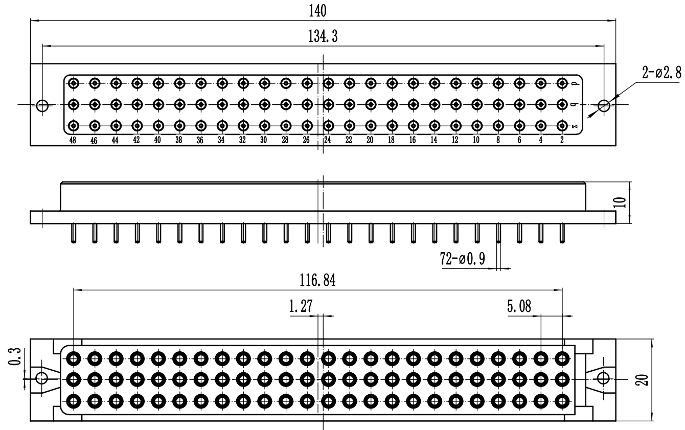
插座安装开孔尺寸(Z)
