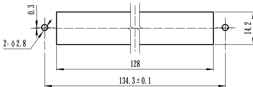
插座安装开孔尺寸
