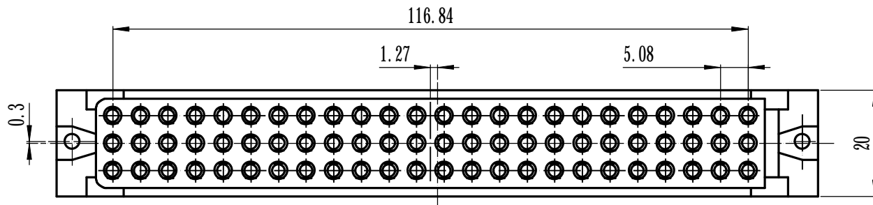
插座安装开孔尺寸
