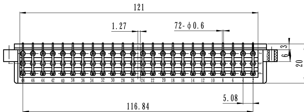
插头推荐安装开孔尺寸
