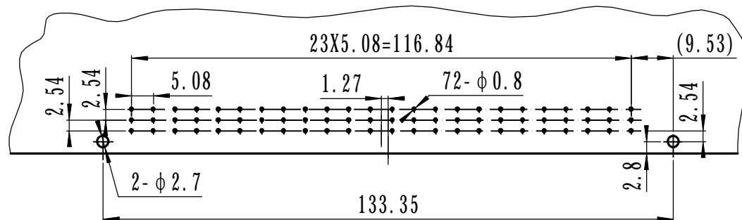
插头推荐安装开孔尺寸
