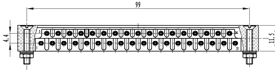
插头安装开孔尺寸
