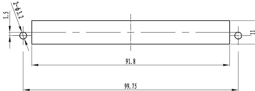
插头安装开孔尺寸
