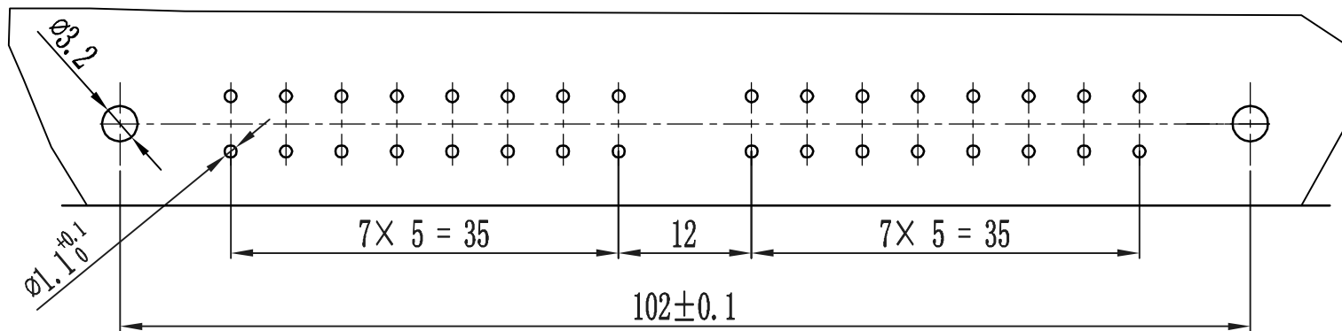
插座安装开孔尺寸
