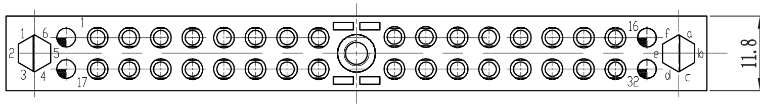
插座安装开孔尺寸
