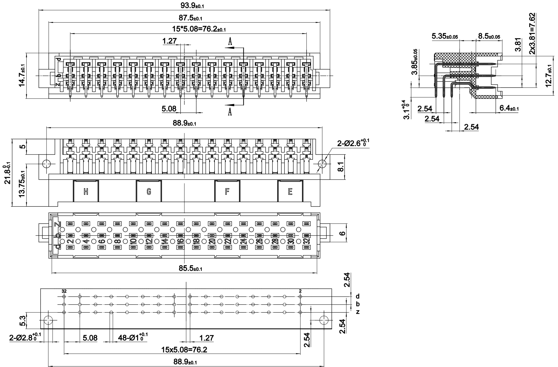
PC板安装孔尺寸
