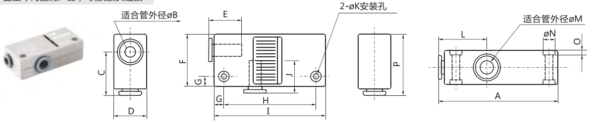
盒型 (内置消声器)-快换接头连接
