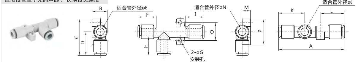
直接接管型 (无消声器)-快换接头连接
