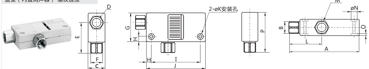
盒型 (内置消声器)-螺纹连接
