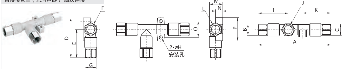
直接接管型 (无消声器)-螺纹连接
