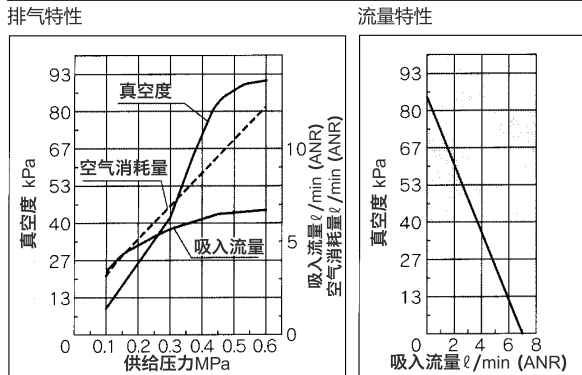
PZU05S 最高真空度: 85kPa
