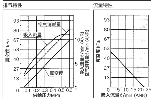
PZU07L 最高真空度: 48kPa
