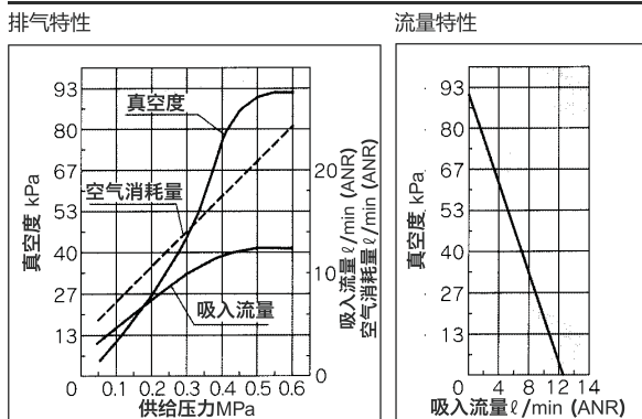
PZU07S 最高真空度: 85kPa
