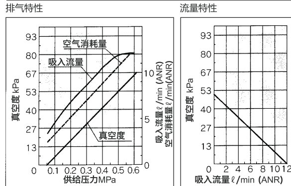
PZU05L 最高真空度: 48kPa
