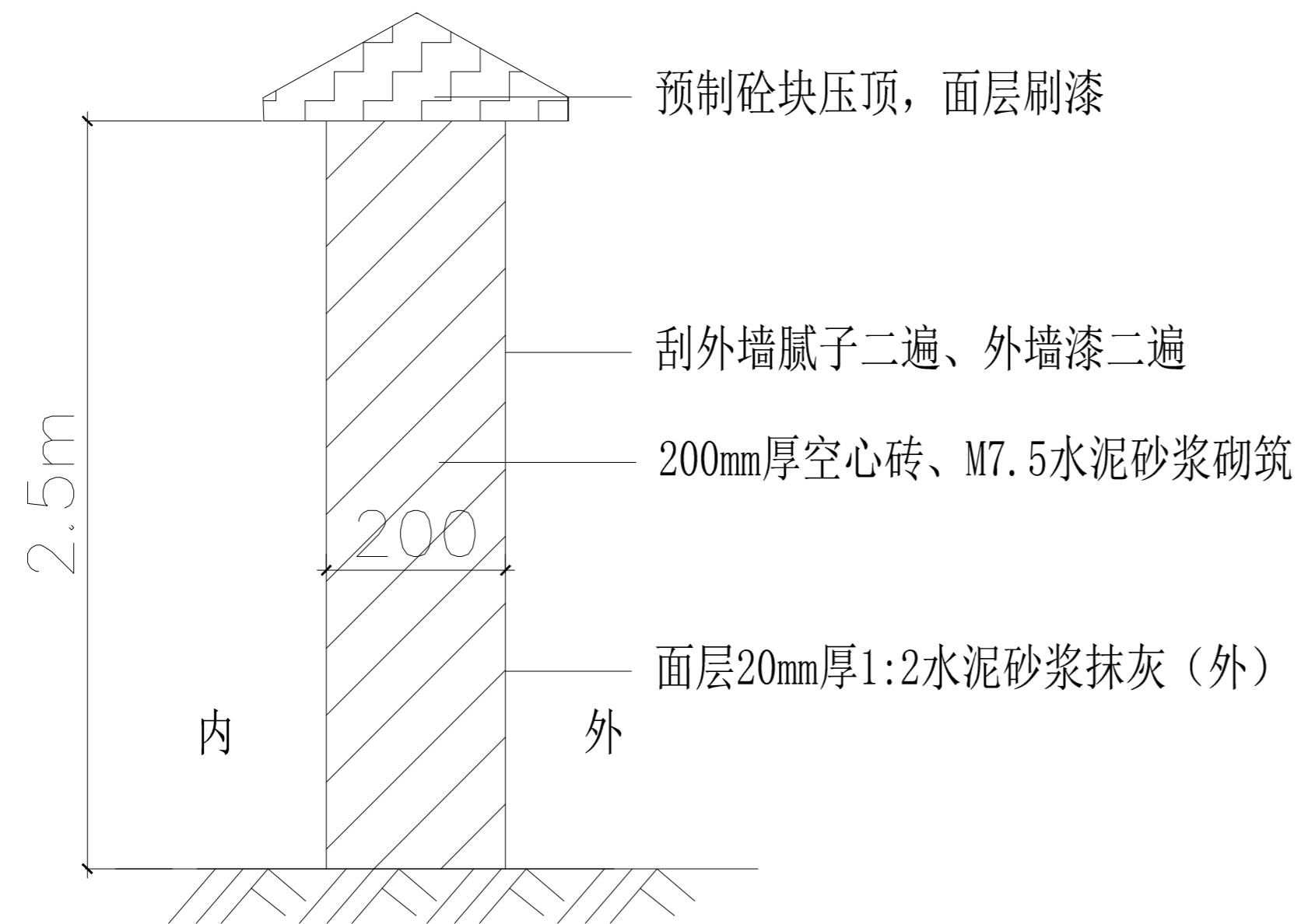
围墙剖面图
