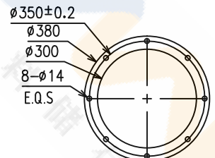
出料口法兰 Discharge Flange
