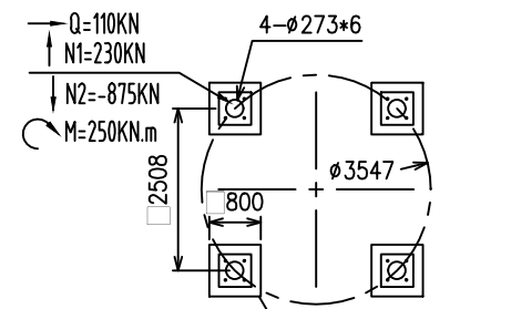
支腿布置示意图 Layout of leg
