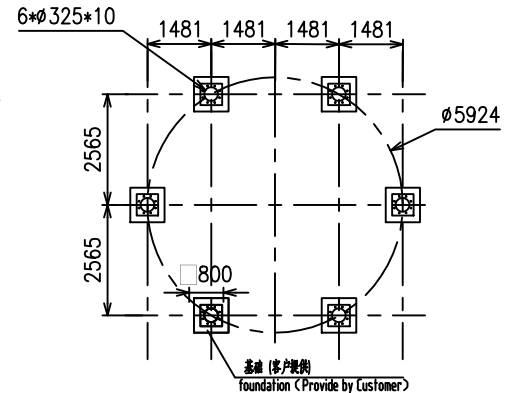
支腿布置示意图
