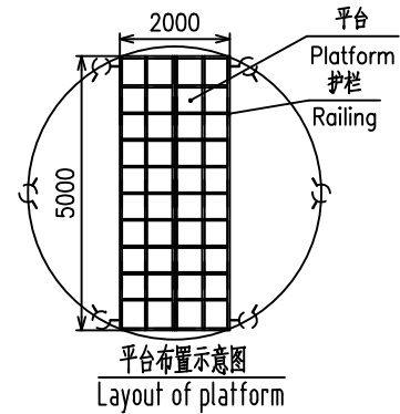
平台布置示意图 Layout of platform
