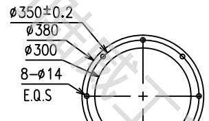
出料口法兰 Discharge Flange
