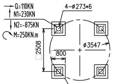
支腿布置示意图 Layout of leg
