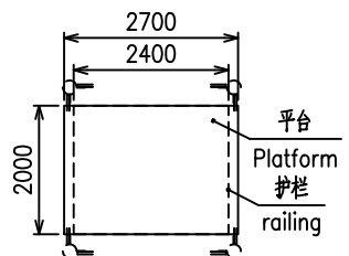
平台布置示意图 Layout of platform
