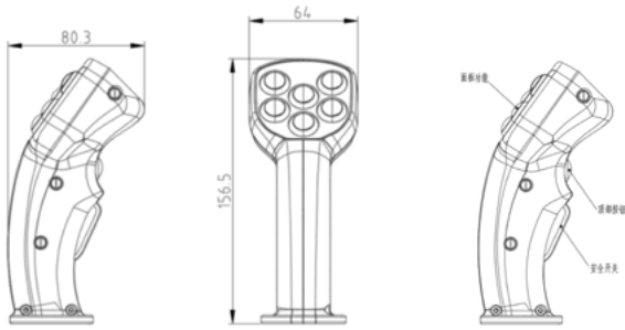
外形尺寸
