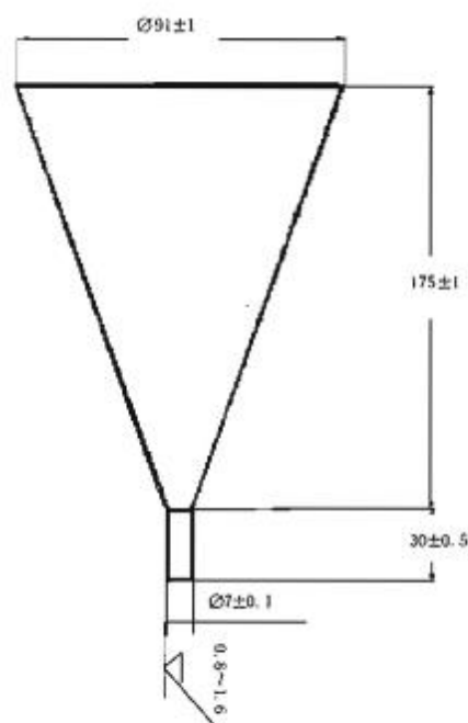
图 1 Marsh 筒示意图
