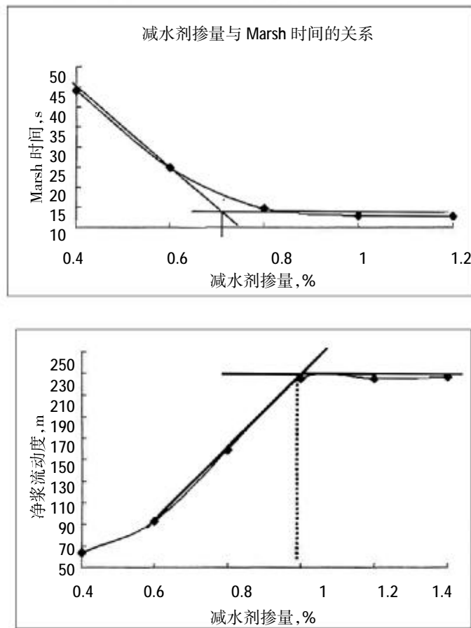
图 1 饱和掺量点确定示意图
