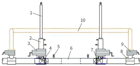
不停输开孔封堵示意图
