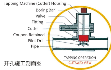
管道不停输带压开孔示意图
