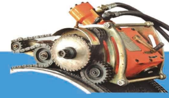
RCH型自爬式液压断管机
