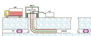
CIPP内衬修复示意图
