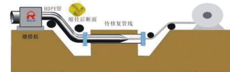
HDPE内衬修复示意图
