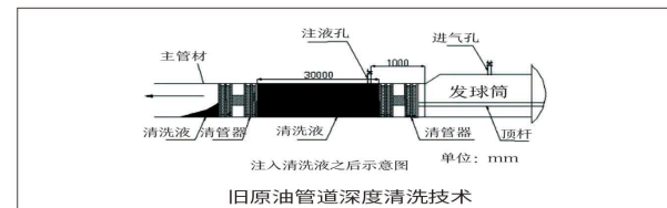
旧原油管道深度清洗技术
