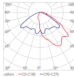
配光曲线
