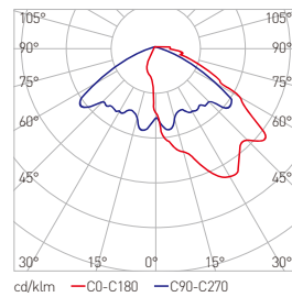
配光曲线
