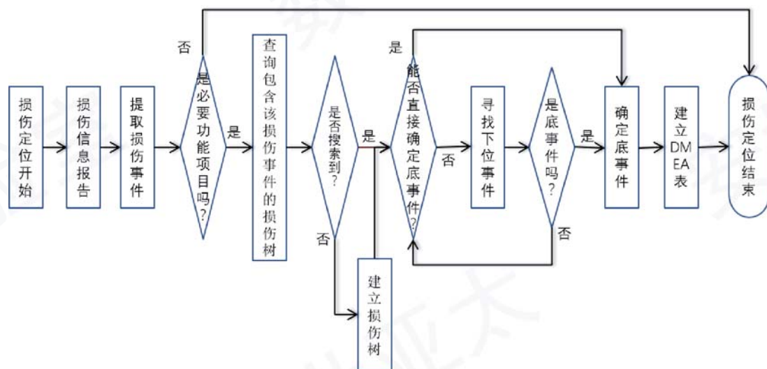
图 56 系统损伤定位分析的基本流程
