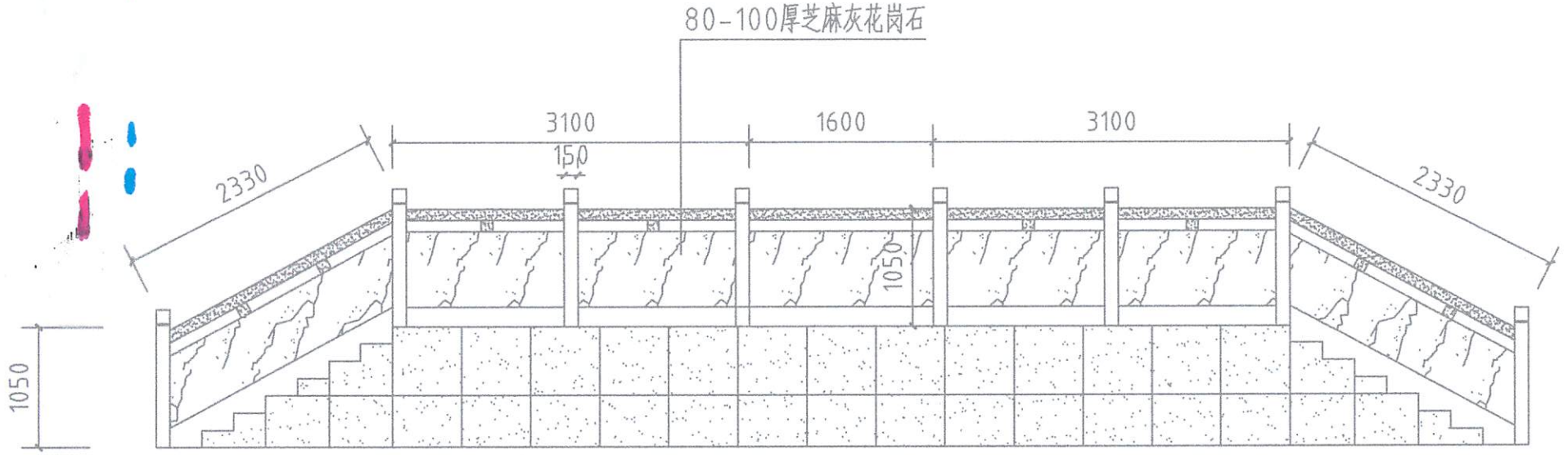
旗台靠操场正立面
