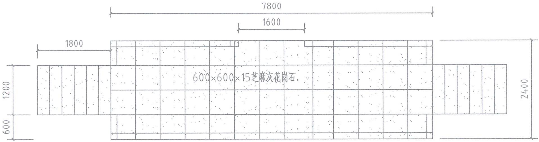
升旗台平面图
