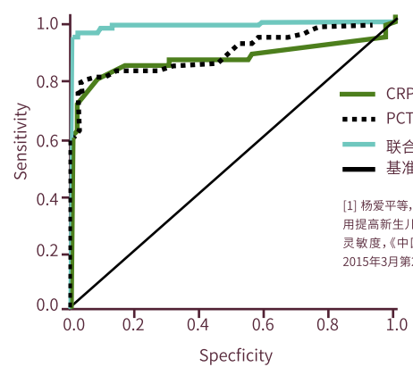
PCT、CRP单独应用及联合应用ROC曲线 [1]
